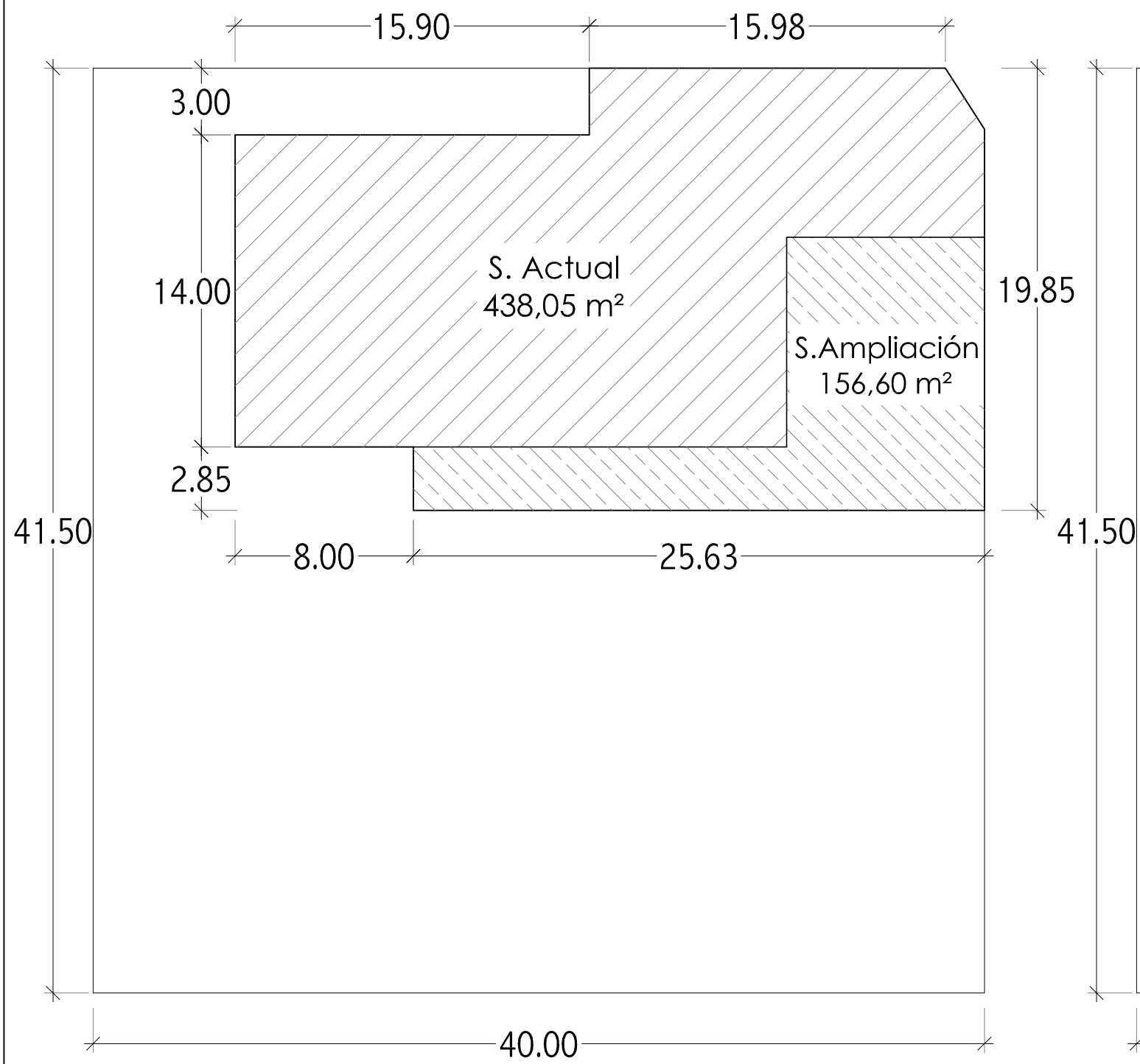
PLANTA BAJA
